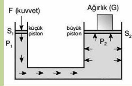
Su cenderesi
