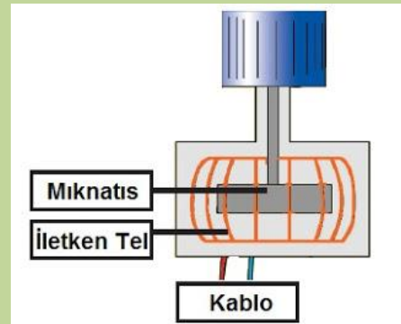
Dinamo Yapısı
