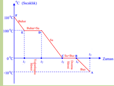
Soğuma Eğrisi
