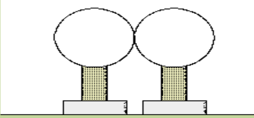
Etki ile elektriklenme - 2
