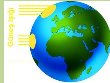
Birim Yüzeye Düşen Işın
