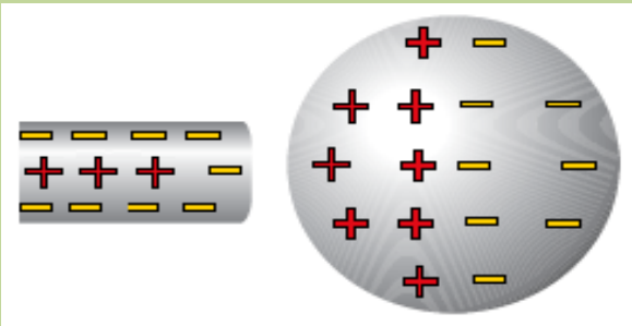
Küre etki ile elektriklenir.
