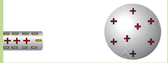
Küre pozitif yükle yüklenir.
