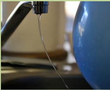
Elektrikleşmiş balon musluktan akan suyu çeker
