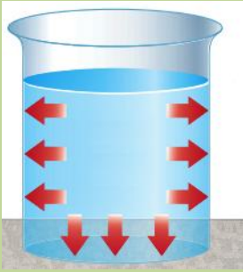
Sıvı Basıncı
