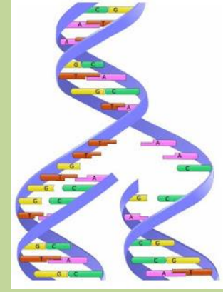
DNA'nın kendini eşlemesi
