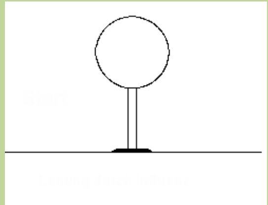
Etki ile elektriklenme
